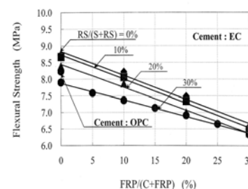
図B ピッチー炭素短繊維補強セメント系複合材料 (ピッチーCFRC)の曲げ強度に及ぼす微粉末化廃 FRP置換率の影響 (EC:エコセメント、OPC:普通 ポルトランドセメント) (EC90%/微粉末化廃 FRP10%で物質・材料効率が10%向上)
